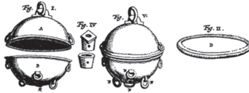
Zuspumpes Experiment mit Guericke's Magdeburger Halbkugeln. Hollnische aus: Otto von Guericke's Experimenta. Amsterdam 1672.
