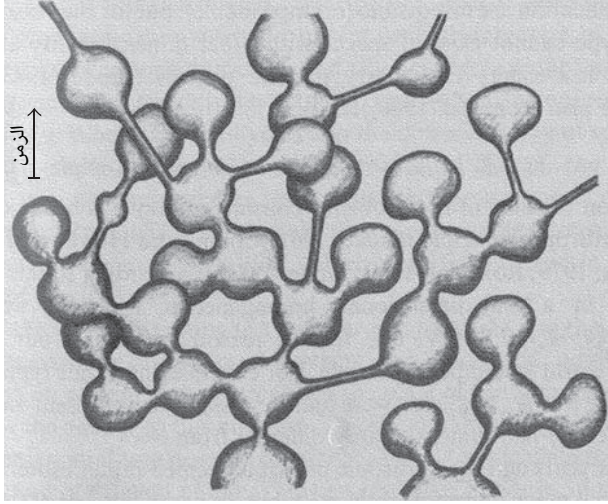
شكل ٨-٢: زبد الزمكان. إحدى الأفكار المرتبطة بالجاذبية الكمية تقضي بأن الزمكان نفسه قد يتحول إلى كتلة هائجة من الفقاعات والأنفاق التي تثب إلى الوجود وتختفي منه على فترات زمنية تناهز زمن بلانك.
