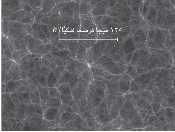
شكل ٧-١: المحاكاة الخاصة بتوزيع المادة في الكون المتمدد الموصوف في النص. هذا يتوافق إلى حدٍ بعيد مع التوزيع المرصود للمجرات.
