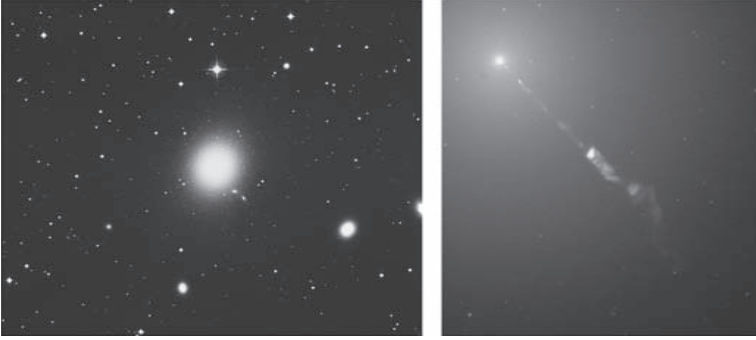
شكل ٧-٢: ثقب أسود نشط. التيار المندفع من مركز المجرة M87 يحركه ثقب أسود، ورغم ظهور التيار بالكاد للعيان في صورة فوتوغرافية ضوئية (إلى اليسار)، فإنه يظهر على نحو أكثر وضوحاً بكثير في الصورة الملتقطة بالأشعة تحت الحمراء (إلى اليمين).
