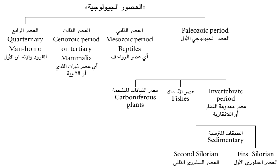
شكل ١٠-١: العصور الجيولوجية.
